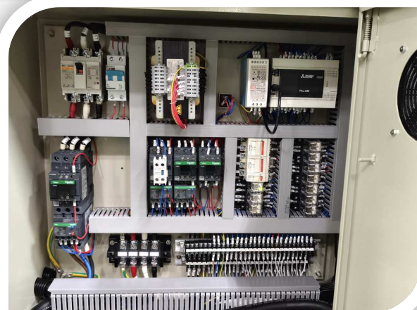
PLC控制/DC-24V 低電壓
